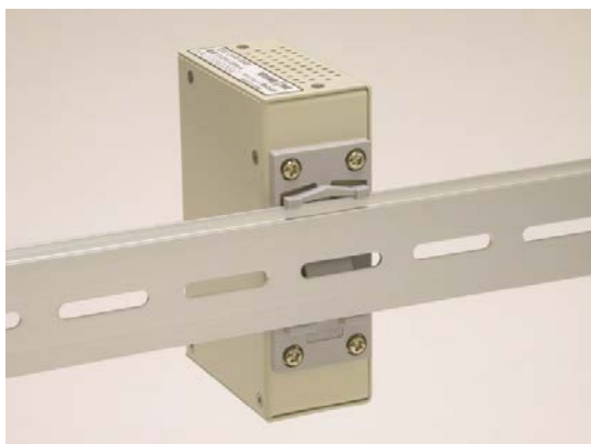
図 13 DIN レール取付具の取付け
