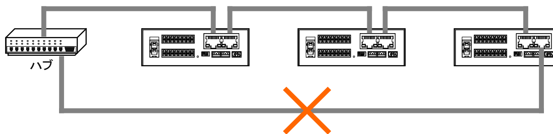
図 23 ループ接続の禁止
