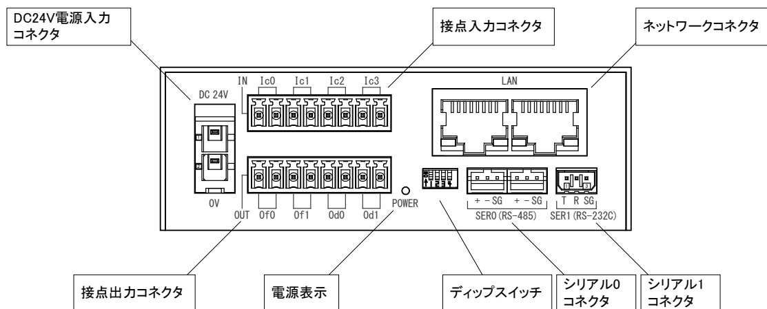
図 11 LANX-I0404 各部の名称
