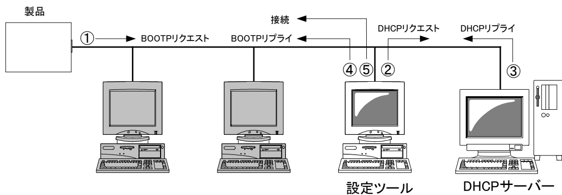
図 36 自動取得した IP の割り当て
