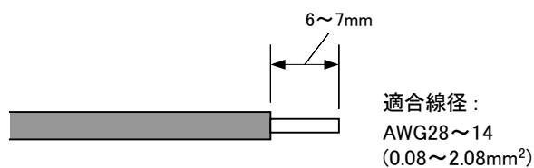
図 15 電線の加工
