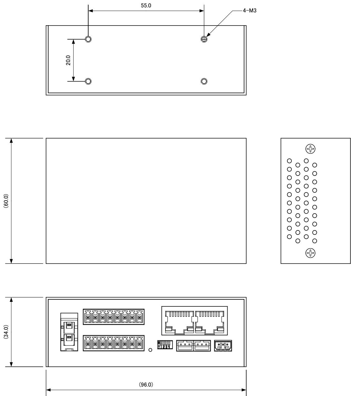
图 9 外形寸法图
