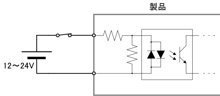
図 25 接点入力の接続例
