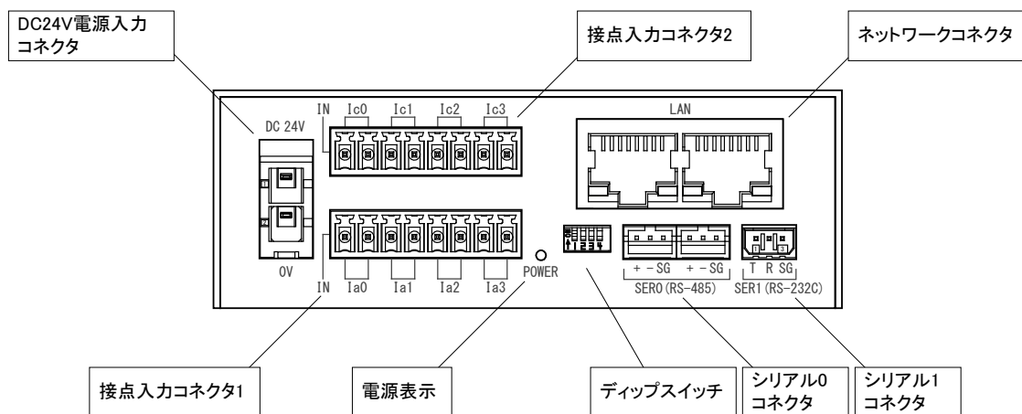
図 10 LANX-I0800 各部の名称
