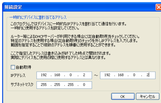
図 19 接続設定画面
